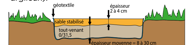
Support et lit de sable
