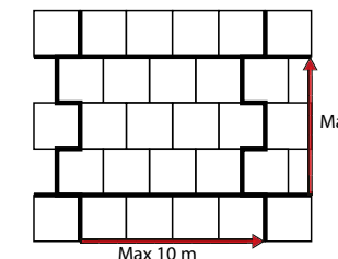
Distances maximales entre les joints de fractionnement.
