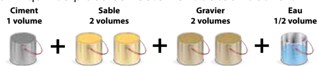
Formule de béton type pour les fondations
